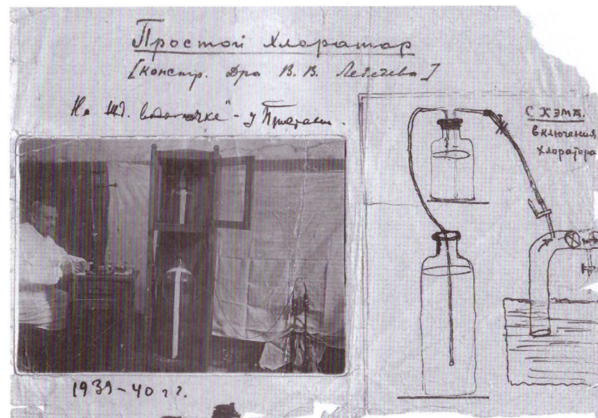
Простой хлоратор конструкции В.В. Лебедева на железнодорожной водопроводке у пристани. Фотография и схема. 1939—1940 годы
