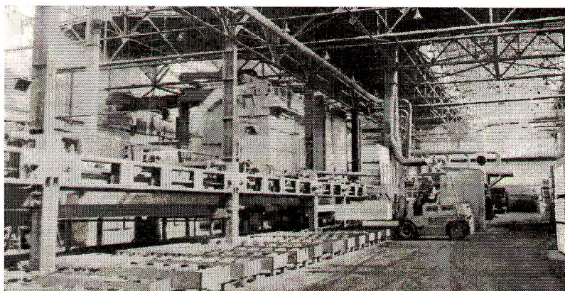
Линия отделки цеха ДСП
