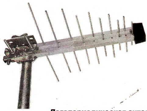
Логопериодическая антенна
