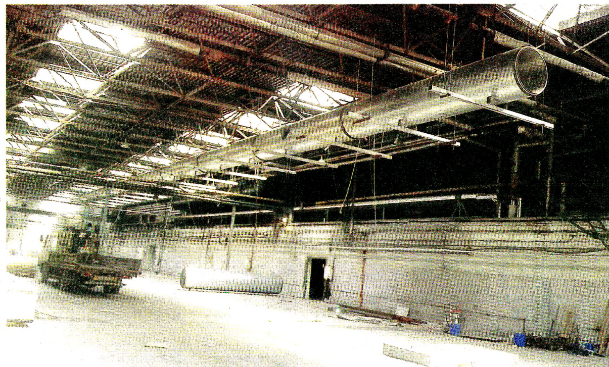
Монтаж воздухопроводов в цехе импрегнирования
