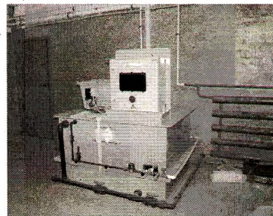
Узел приготовления и дозирования извести
