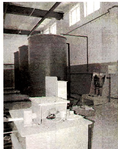
Насосная группа и емкости для коагулянта
