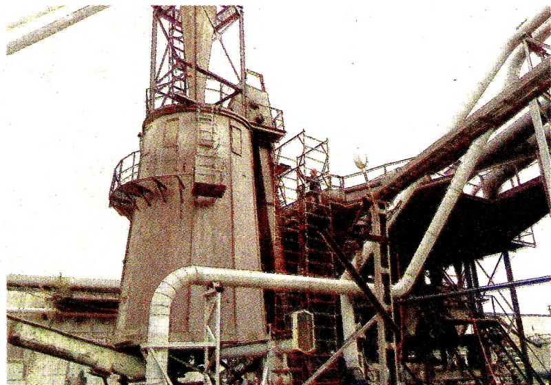
Заменены воздуховоды системы аспирации шлифовальной пыли
