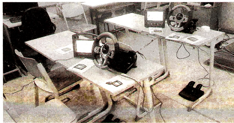
Тренажёры системы параллельного вождения «Агронавигатор»
